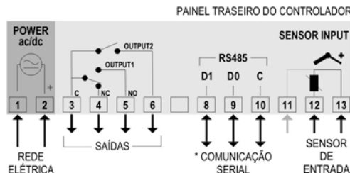
Fig. 01 – Conexões mostradas na etiqueta do controlador
