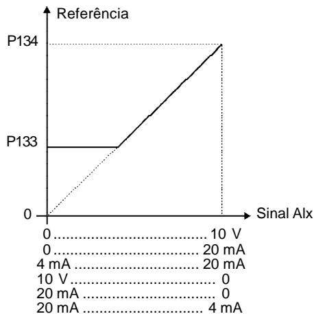
Figura 6.28 b) - Atuação das Entradas Analógicas
