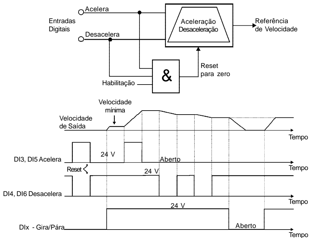
Figura 6.37 k) a m) (cont.) - Detalhes sobre funcionamento das funções das entradas digitais
