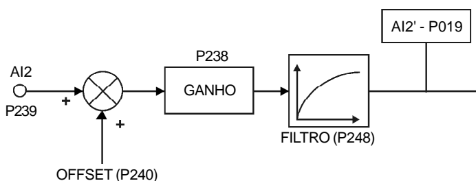
Figura 6.30 - Blocodiagrama da entrada Analógica AI2
