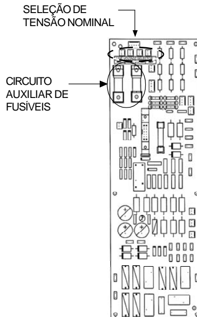
Figura 3.8 a) e b) - Seleção da Tensão Nominal nos Cartões LVS1, CIP2, LVS2 e CIP3
