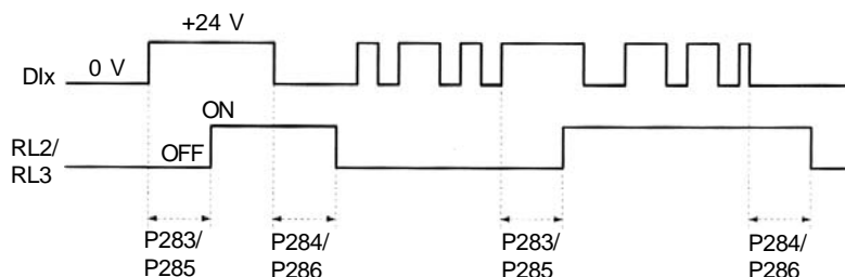
Figura 6.36 - Funcionamento da função temporizador RL2 e RL3
