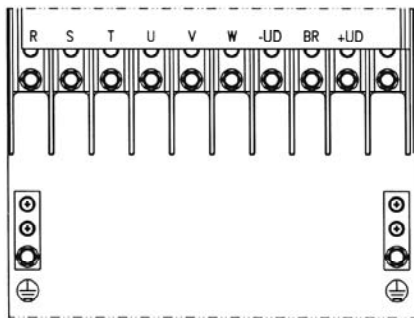
e) Modelo da mecânica 7 (500-600 V)
