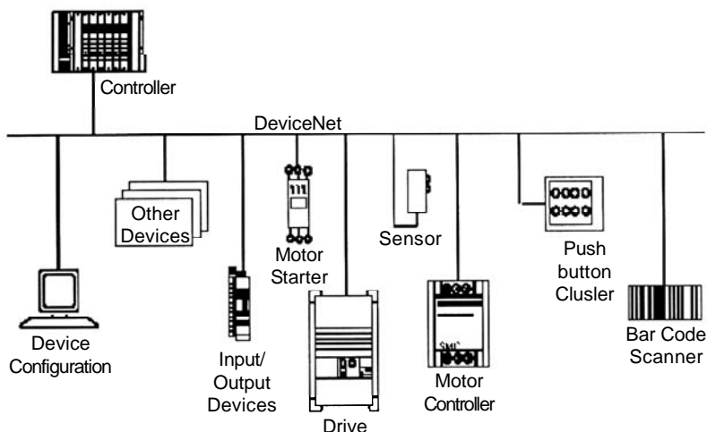
Figura 8.41 - Rede DeviceNet
