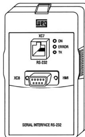
Figura 8.18 - Módulo RS-232
