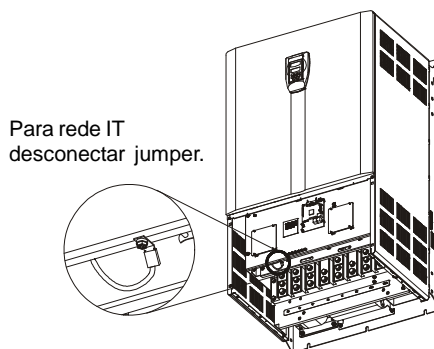
Figura 3.11 a) a g) - Posicionamento do jumper para desconexão do varistor e capacitor contra o terra - necessário apenas em alguns modelos de inversores quando o mesmo for conectado a uma rede IT
