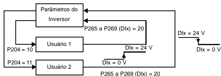
Figura 6.35 - Detalhes sobre o funcionamento da função carrega usuário via Dlx
