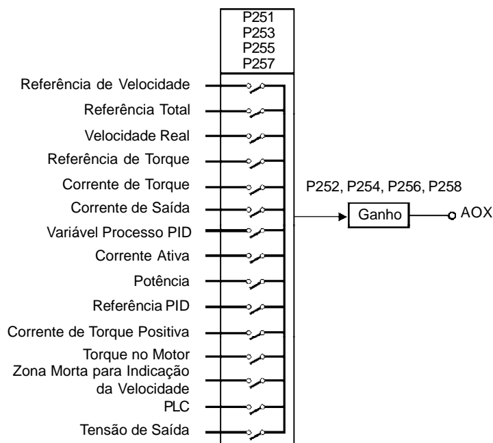
Figura 6.31 - Blocodiagrama das Saídas Analógicas
