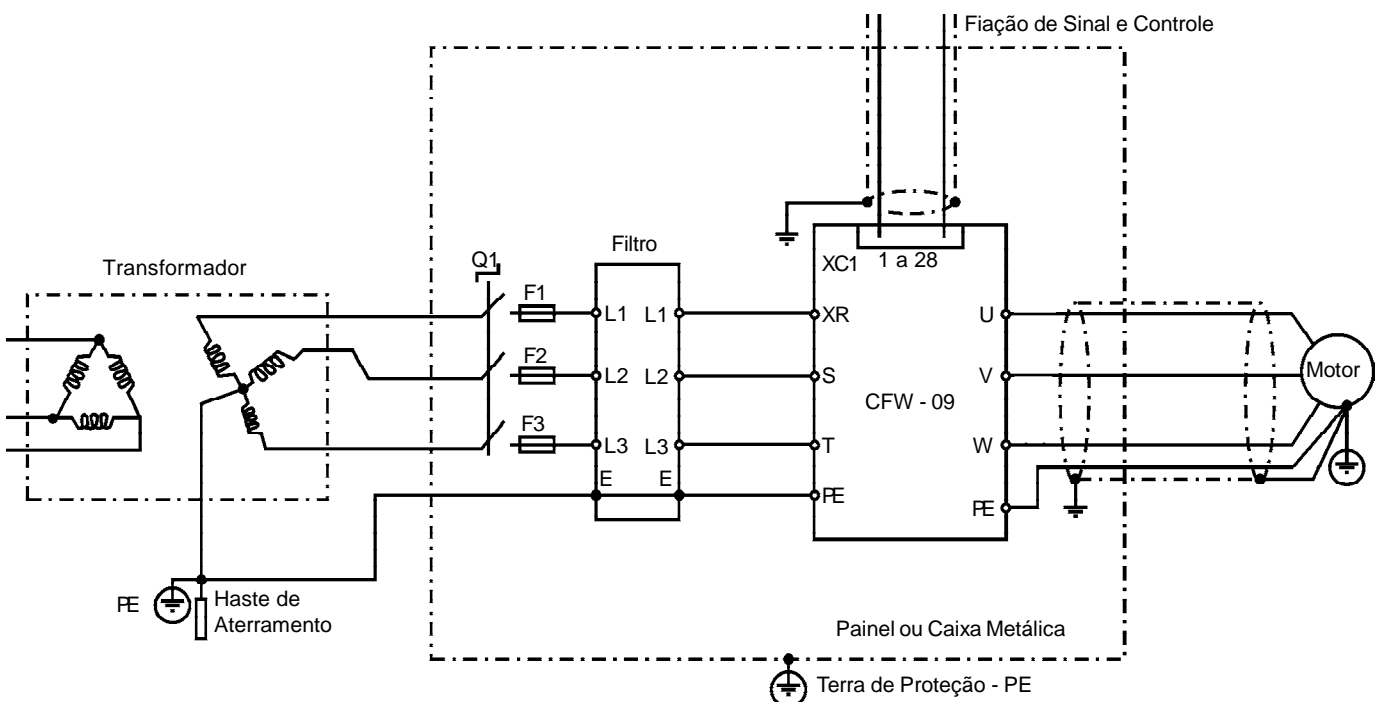
Figura 3.18 - Conexão dos filtros de EMC EPCOS em inversores de frequência CFW-09
