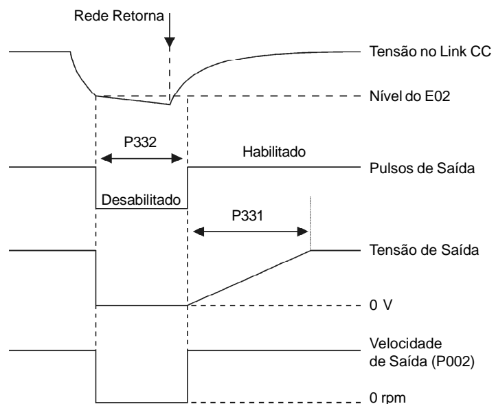
Figura 6.44 a) - Atuação do Ride-Through (rede retorna antes do tempo ajustado em P332) em Modo V/F
