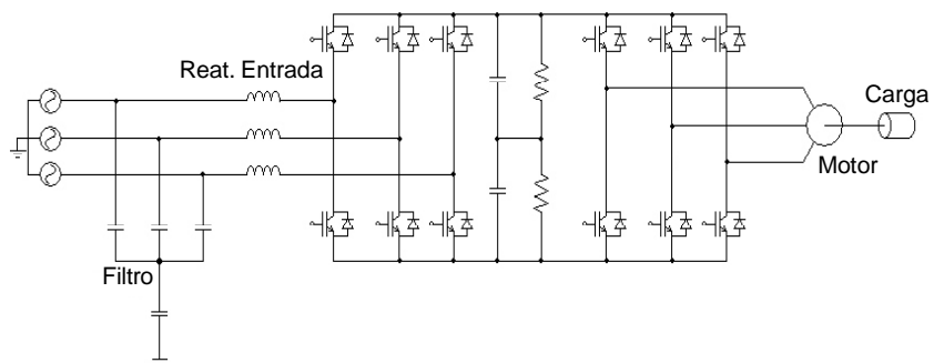
Figura 8.58 - Esquema simplificado de um acionamento com o CFW-09 RB
