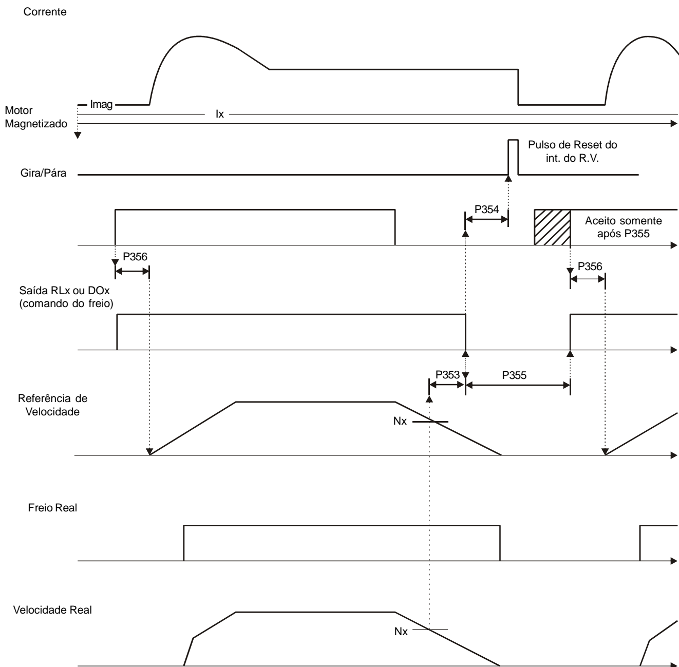
Figura 6.39 s) (cont.) - Detalhes do funcionamento das funções das saídas digitais e a relés
