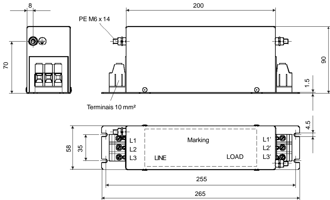
Figura 3.20 c) e d) - Filtros EMC para os inversores de frequência da linha CFW-09 [dimensões em mm (in)]
