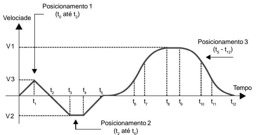
Figura 8.60 - Trajetória com utilização da placa PLC
