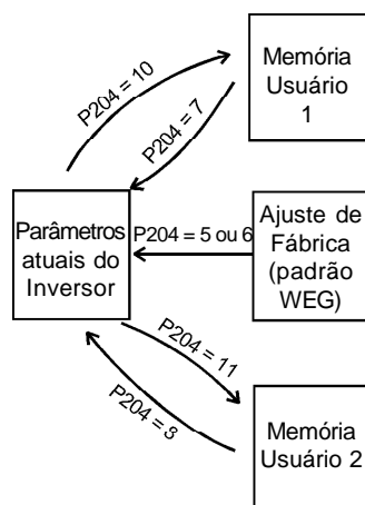
Figura 6.23 - Transferência de parâmetros
