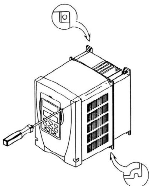
Figura 3.3 a) e b) - Procedimento de instalação do CFW-09 em superfície
