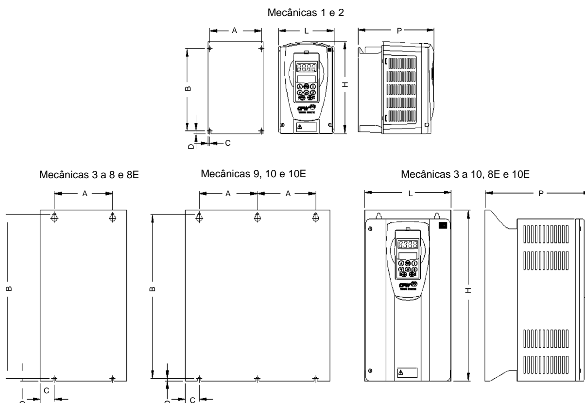
Figura 3.1 - Dimensional para fixação do CFW-09
