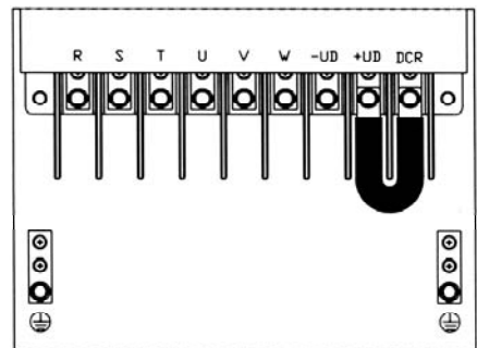
f) Modelo da mecânica 8 (380-480 V)
