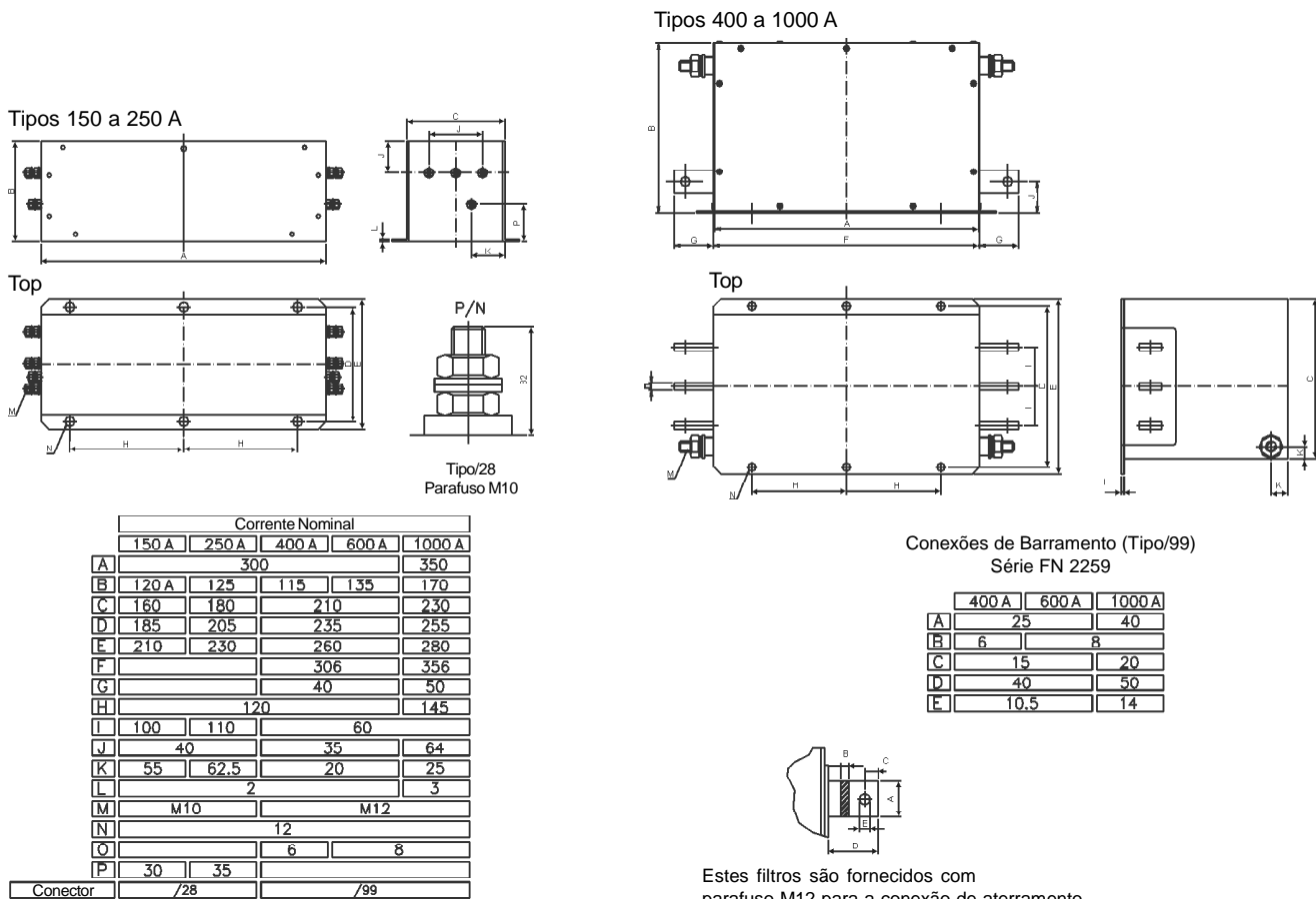
Figura 3.20 r) - Filtros EMC para os inversores de frequência da linha CFW-09 [dimensões em mm (in)]
