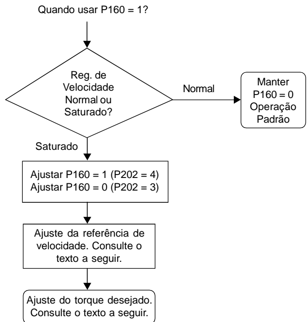
Figura 6.19 - Controle de Torque
