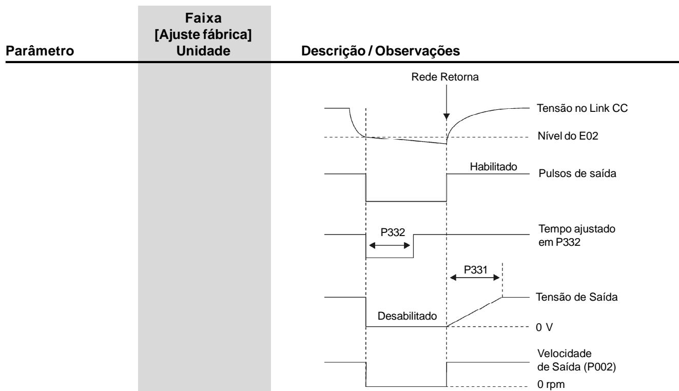
Figura 6.44 b) - Atuação do Ride-Through (rede retorna depois do tempo ajustado em P332, mas antes de 2 s para P332 \leq 1 s ou antes de 2 \times P332 para P332 > 1 s) em Modo V/F
