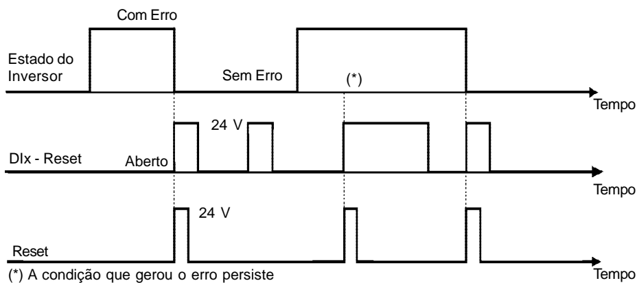
Figura 6.37 h) a j) (cont.) - Detalhes sobre funcionamento das funções das entradas digitais
