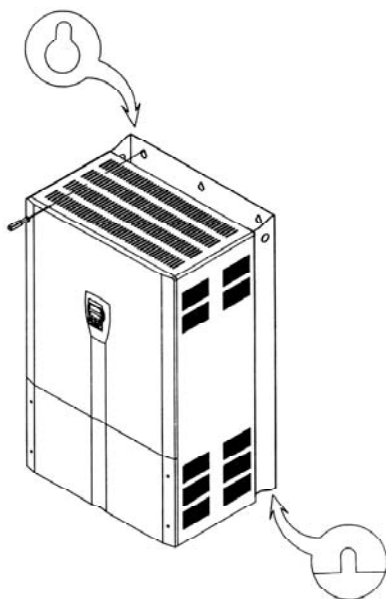
Figura 3.3 c) e d) - Procedimento de instalação do CFW-09 em superfície
