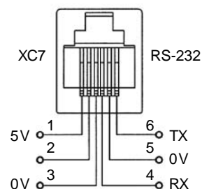
Figura 8.50 - Descrição sinais do conector XC7 (RJ12)
