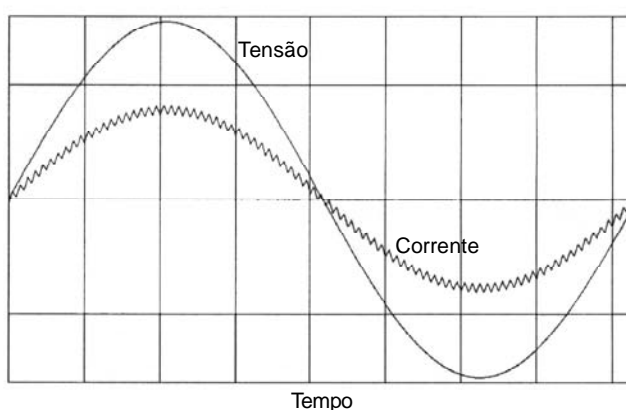
Figura 8.59 a) - Funcionamento durante a motorização
