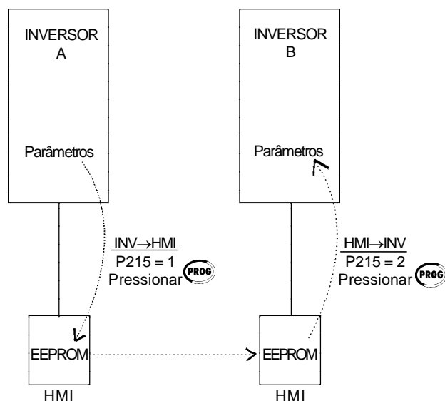
Figura 6.24 - Cópia dos Parâmetros do "Inversor A" para o "Inversor B"
