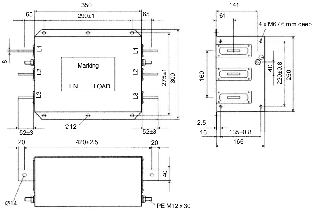
Figura 3.20 k) e l) - Filtros EMC para os inversores de frequência da linha CFW-09 [dimensões em mm (in)]
