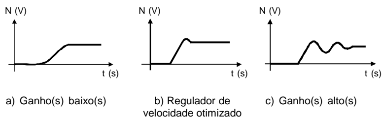
Figura 6.20 - Tipos de resposta do Regulador de Velocidade
