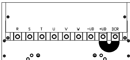
g) Modelo das mecânicas 9 e 10 (380-480 V)
