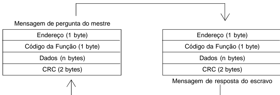
Figura 8.51 - Estrutura dos telegramas
