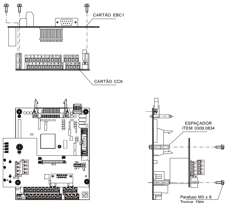
Figura 8.10 - Procedimento de Instalação do cartão EBC1
