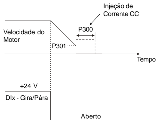
Figura 6.40 a) e b) - Atuação da Frenagem CC no Bloqueio por Rampa (via desabilita por rampa)
