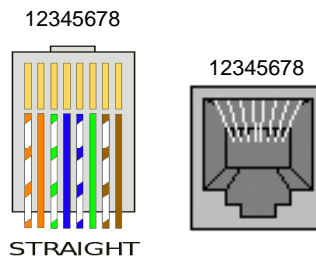
Figura 8.45 a) e b) - Padrões para cabos Ethernet direto (Straight-Through)
