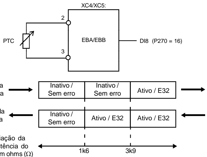
Figura 6.33 - DI8 como PTC
