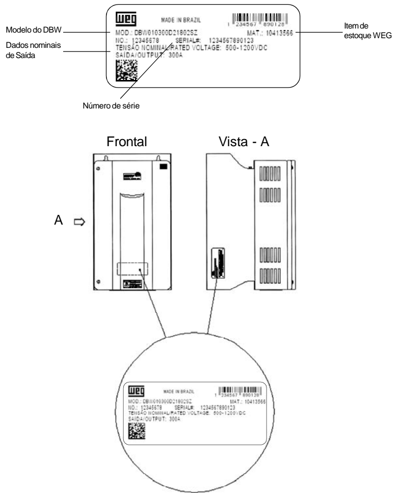
Figura 8.23 - Etiqueta de identificação
