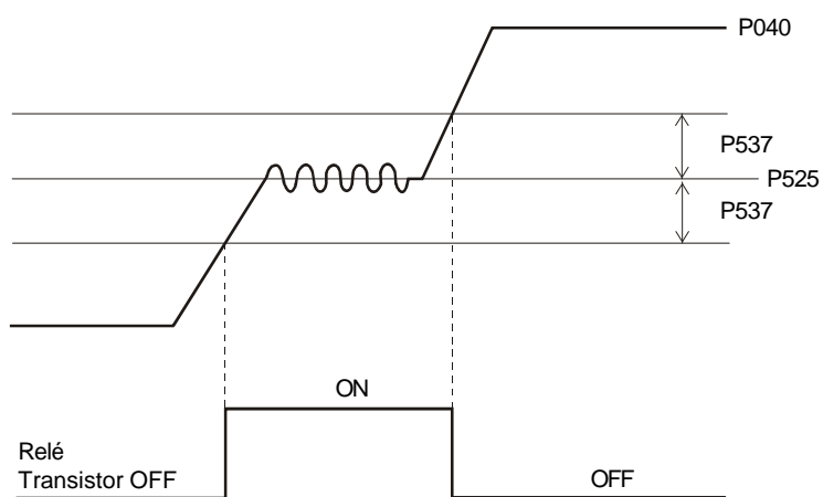
Figura 6.39 t) a v) (cont.) - Detalhes do funcionamento das funções das saídas digitais e a relés
