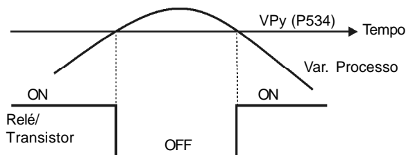
Figura 6.39 i) a p) (cont.) - Detalhes do funcionamento das funções das saídas digitais e a relés
