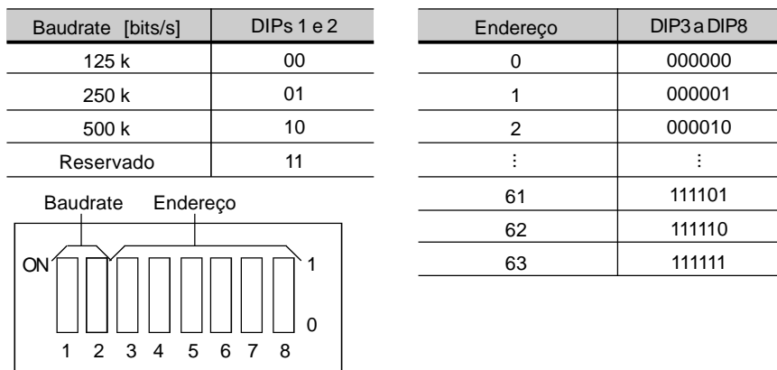
Figura 8.42 - Configuração do baudrate e endereço para DeviceNet
