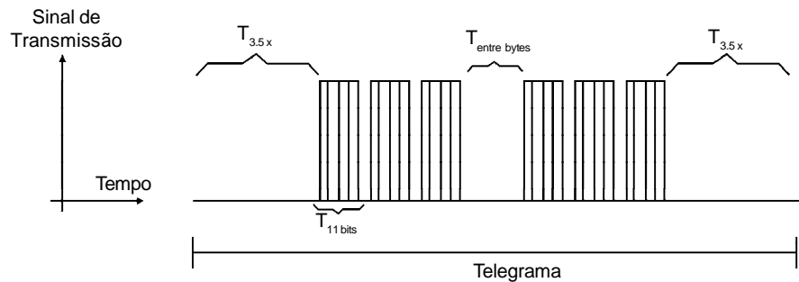
Figura 8.52 - Tempos envolvidos durante a comunicação de um telegrama
