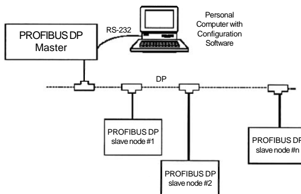
Figura 8.39- Rede Profibus DP
