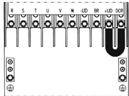
d) Modelo da mecânica 6 e 7 (220-230 V e 380-480 V)
