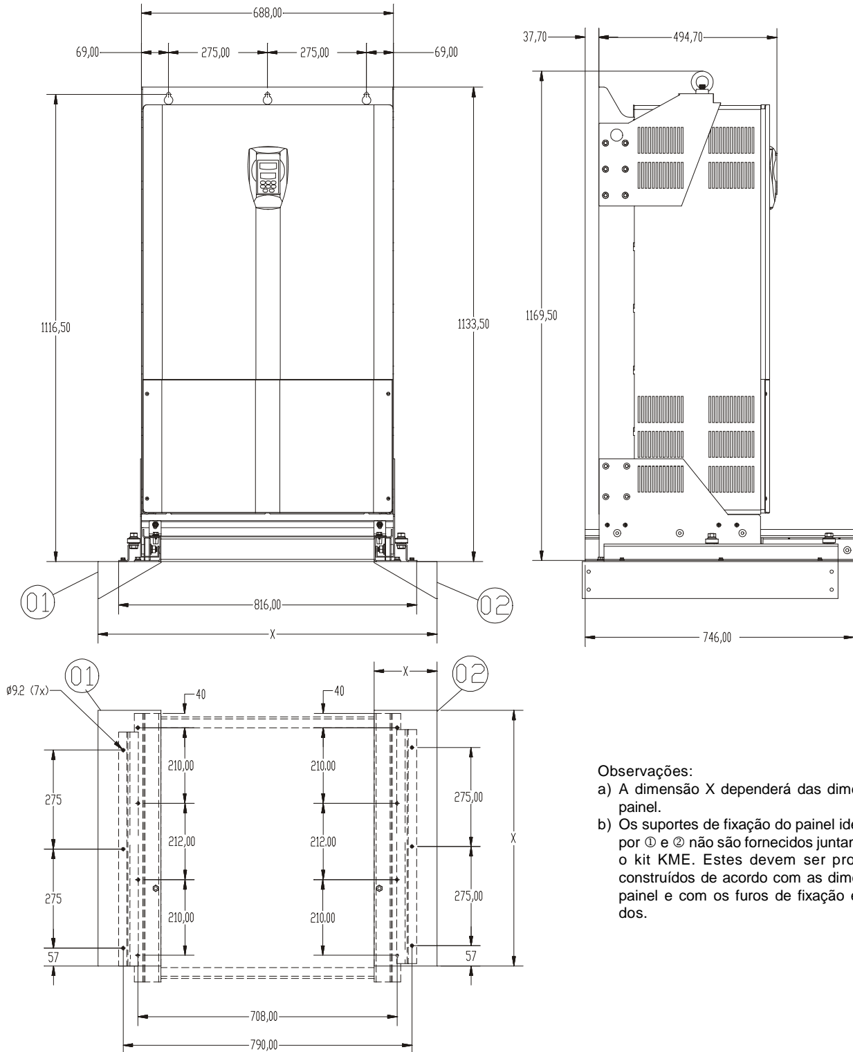
Figura 9.13 - Kit KME - Mecânica 9 - Painel com largura = 800 mm e 1000 mm
