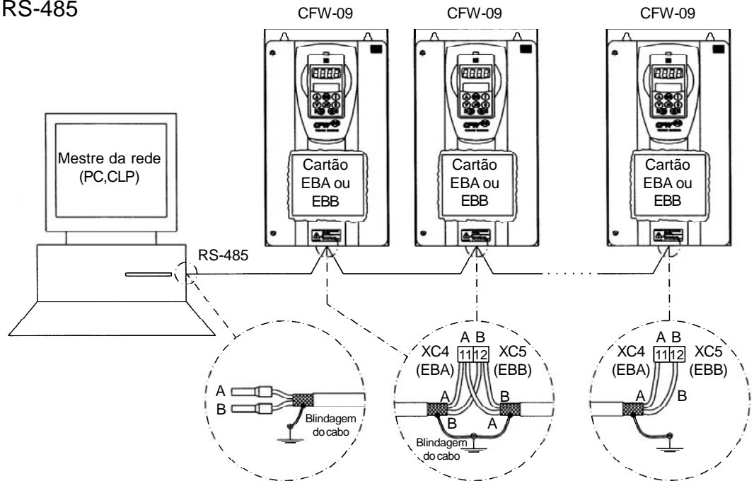
Figura 8.49 - Conexão CFW-09 em rede através da Interface Serial RS-485
