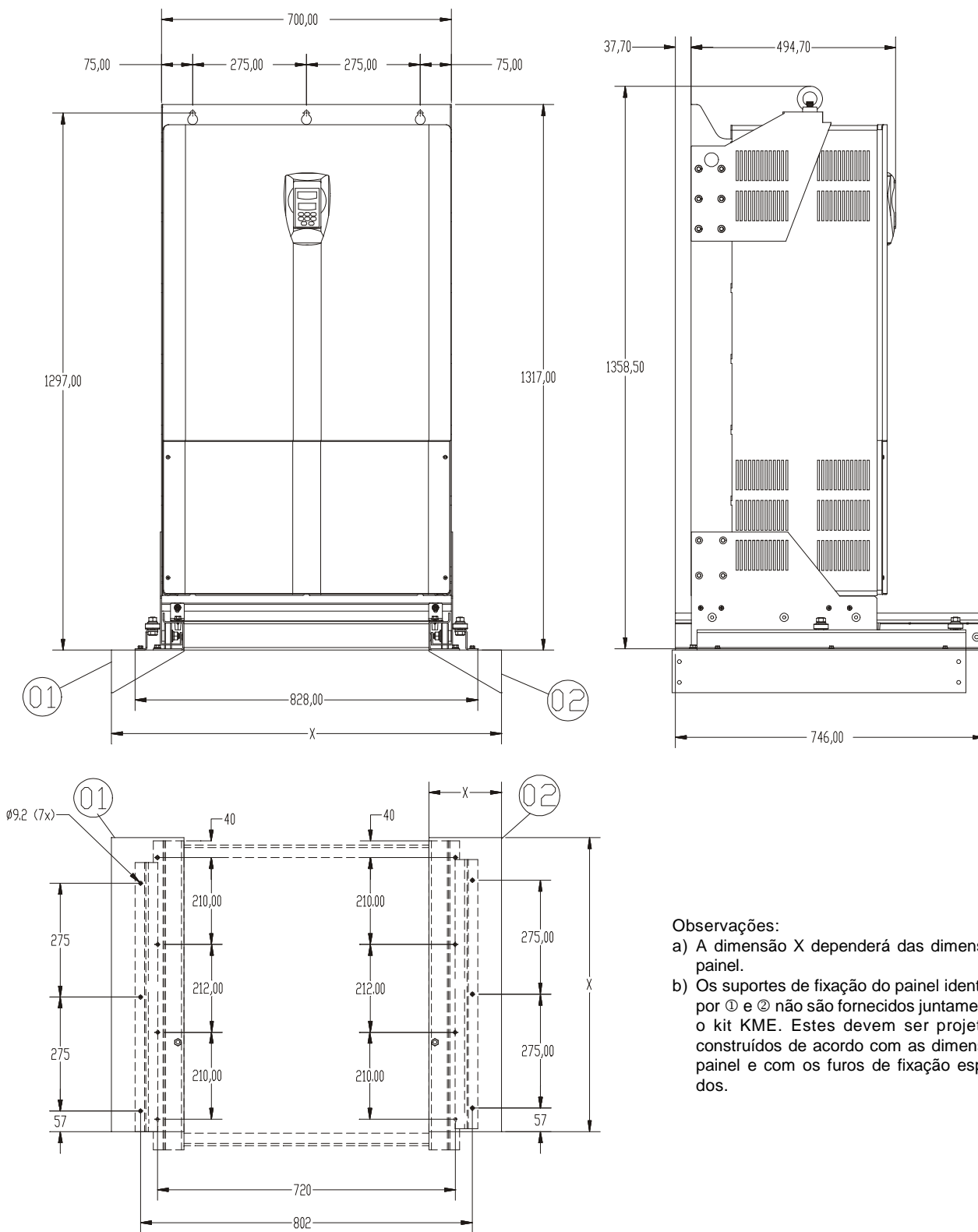
Figura 9.14 a) - Kit KME - Mecânica 10 - Painel com largura 1000 mm
