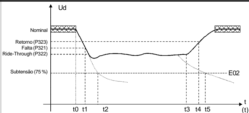
Figura 6.42 - Atuação da Função Ride-Through em Modo Vetorial
