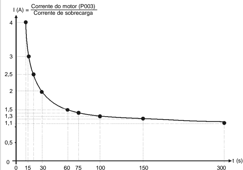
Figura 6.17 – Função Ixt – detecção de sobrecarga
