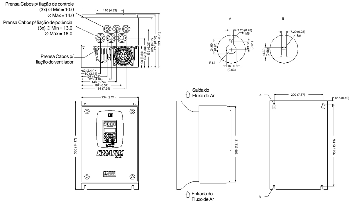
Figura 8.55 - Dados dimensionais em mm (in) - Mecânica 1
