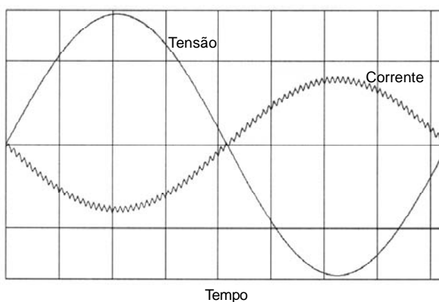
Figura 8.59 b) - Funcionamento durante a frenagem
