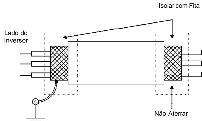
Figura 3.14 - Conexão blindagem
