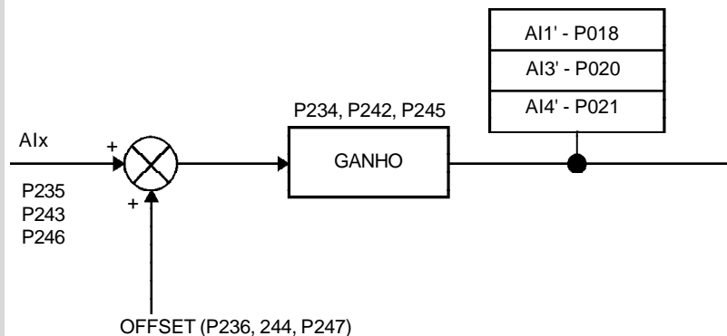
Figura 6.29 - Blocodiagrama das Entradas Analógicas AI1, AI3 e AI4
