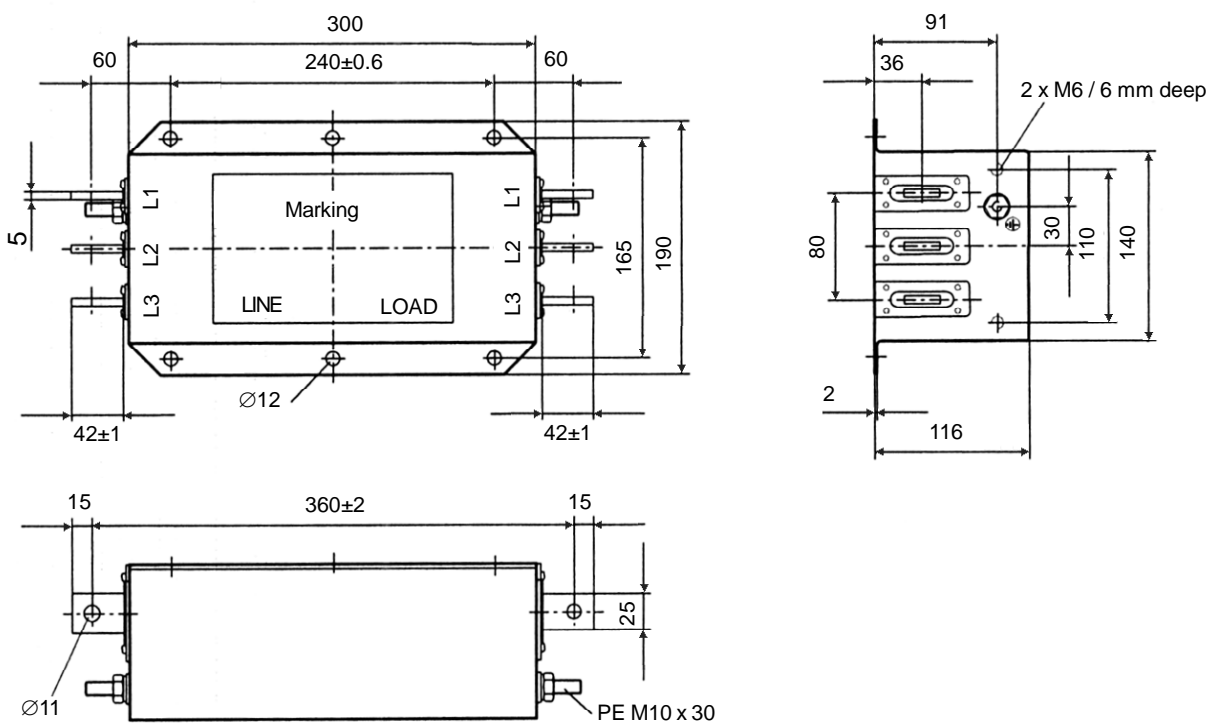
Figura 3.20 m) e n) - Filtros EMC para os inversores de frequência da linha CFW-09 [dimensões em mm (in)]
