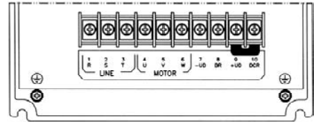
b) Modelo da mecânica 2
