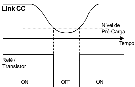
Figura 6.39 i) a p) (cont.) - Detalhes do funcionamento das funções das saídas digitais e a relés
