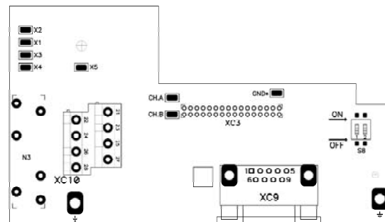
Figura 8.9 - Posição dos elementos de ajuste - cartão EBC
