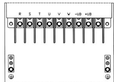
h) Modelo da mecânica 8E (500-690 V e 660-690 V)
