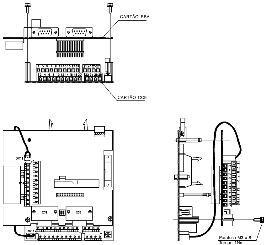
Figura 8.3 - Procedimento de instalação do cartão EBA
