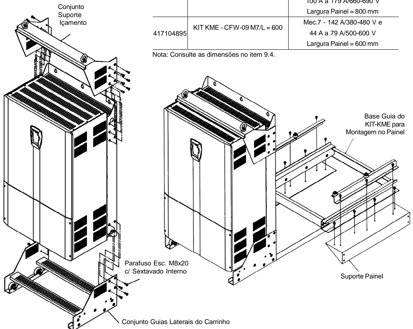
Figura 8.53 - Montagem KIT-KME no inversor
